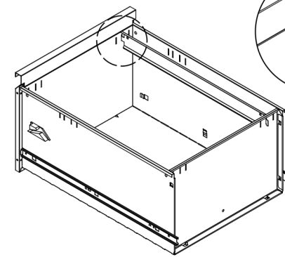
Fastgør ophængsstængerne til skuffepanellerne som vist på billedet.
