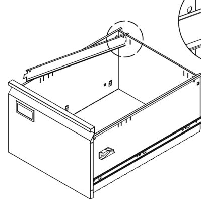
Zamontuj drążki zawieszenia.
