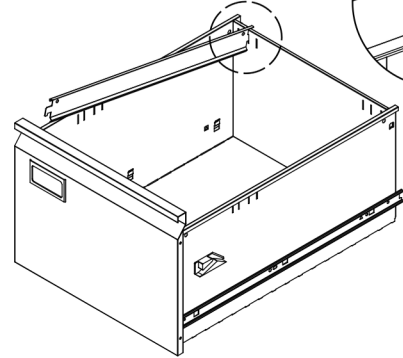
Namontujte závěsné tyče.
