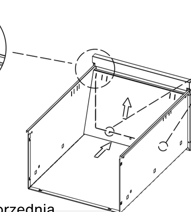
Zamontuj przednią osłonę szuflady zgodnie z rysunkiem.
