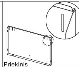
Priekinis stalčiaus dangtelis: 4 vnt.
