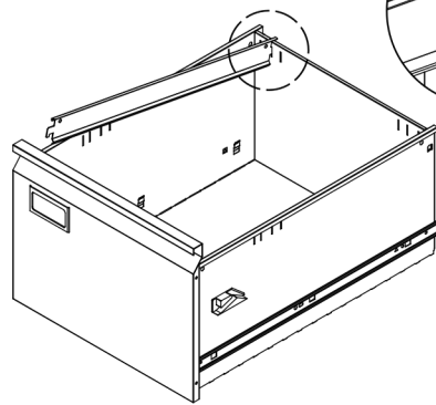
Monter ophængsstængerne.
