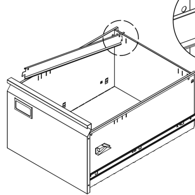
Asenna ripustustangot.
