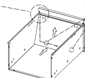
Monter det forreste skuffedæksel som vist på billedet.
