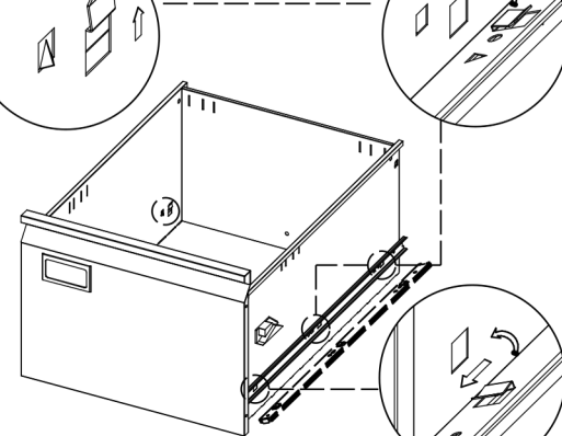
Asenna sisäkiskot.
