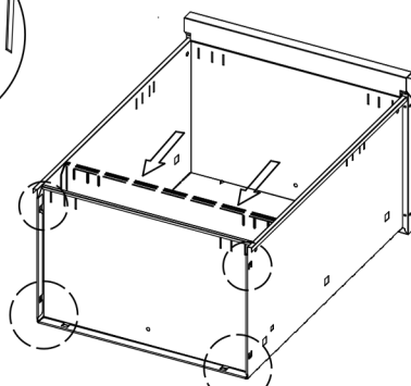
Sumontuokite stalčiaus priekinę plokštę pagal paveikslėlį.
