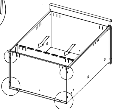
Monter skuffens frontpanel som vist på billedet.
