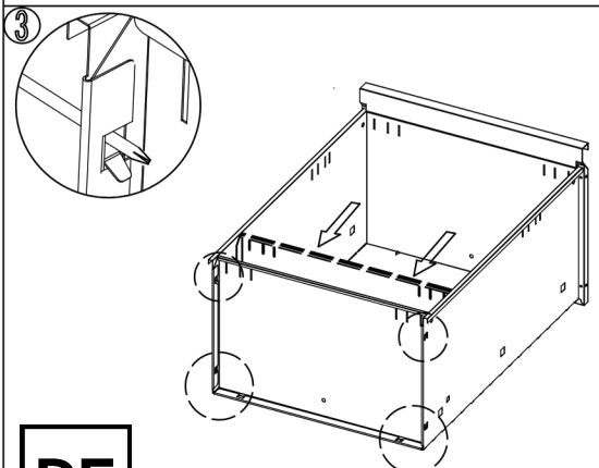
Montieren Sie die Schubladenfront gemäß der Abbildung.
