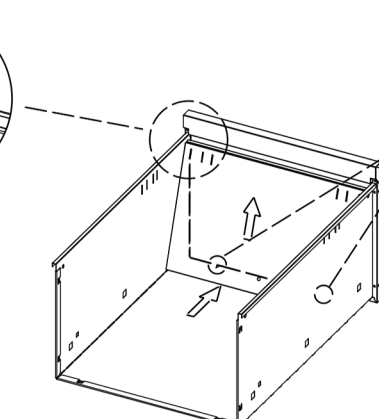
Asenna laatikon etusuojus kuvan mukaisesti.
